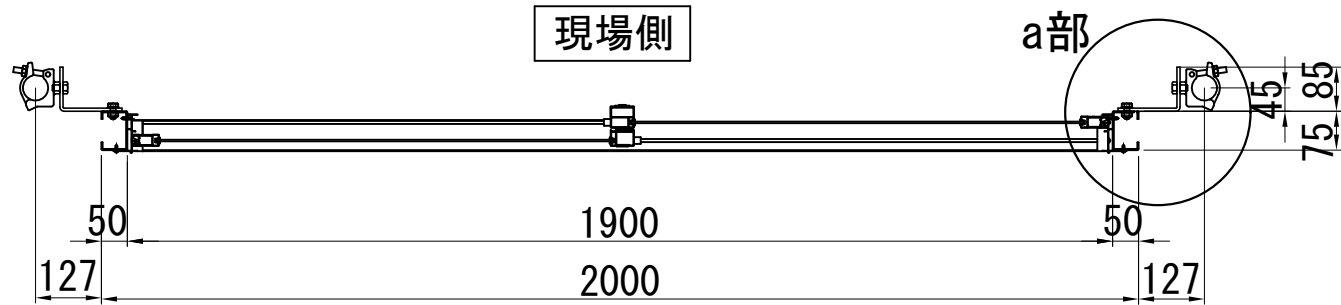
平面图
