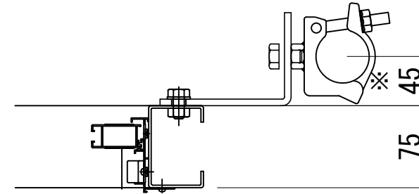
a部詳細
