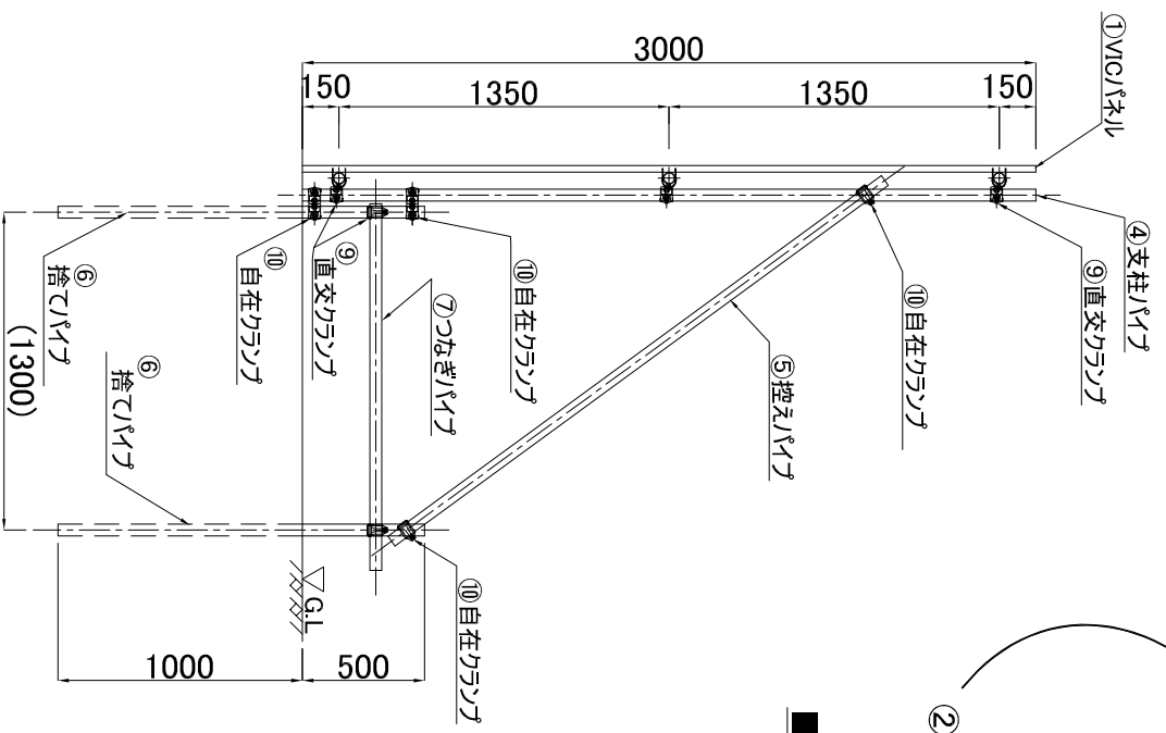
■標準断面図
